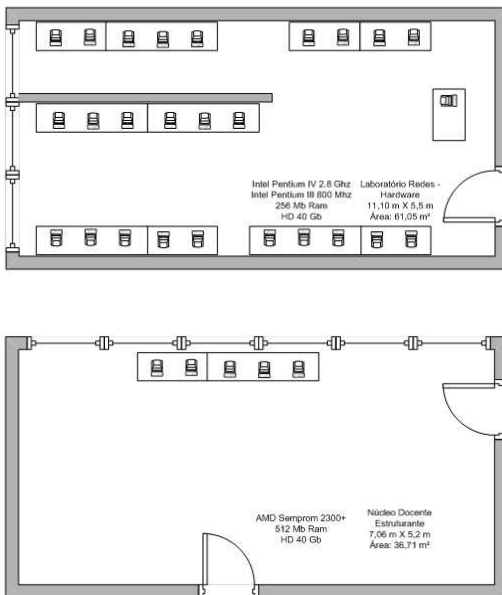
Figura 4.1: Planta simplificada dos laboratórios das Faculdades Integradas Paulista.
